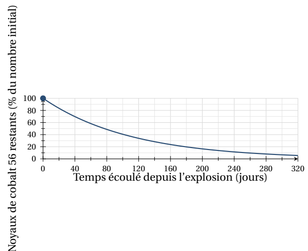
FIGURE 4 – Modèle : décroissance du nombre de noyaux de cobalt 56 formés lors de l'explosion (d'après la luminosité observée de SN 1987A, qui a décru en suivant cette loi entre 4 et 16 mois).
