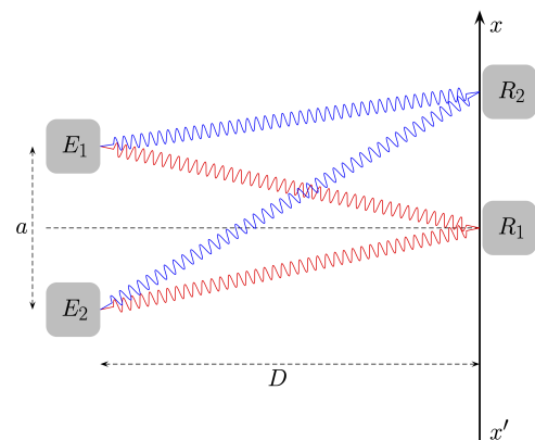
FIGURE 1 – Les interférences vont être observées sur l'écran à droite
